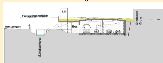
Schnitt C-C (Chileplatz)
